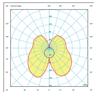
SKYLUM CEILING (SKC): Za namestitev do višine 3 m na hodnikih, s simetrično podolžno porazdelitvijo svetlobe.
