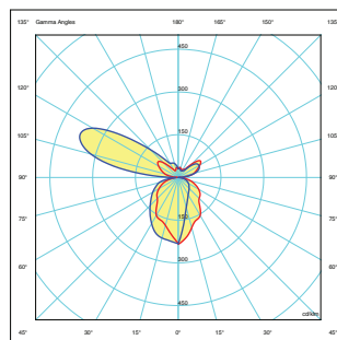
SKY LUM WALL (SKW): Za stensko namestitev do višine 3 m na hodnikih, s posredno in neposredno porazdelitvijo svetlobe.
